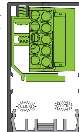
VISTA FRONTALE HERO MINI MODULO SPOT LED KLIMT Hero mini front view Klimt spot LED module
