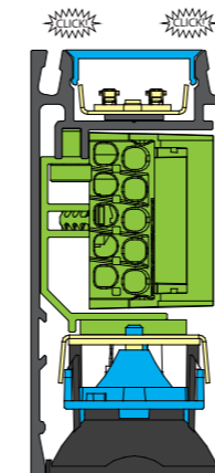
VISTA FRONTALE HERO MINI B MODULO LED MICRO OTTICHE Hero mini front view Micro optics LED module
