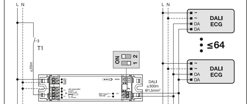
Schema elettrico: modalità PUSH Wiring diagram: TOUCH DIM mode
