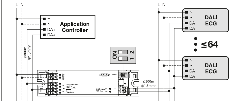
Schema elettrico: modalità DALI Wiring diagram: DALI mode
