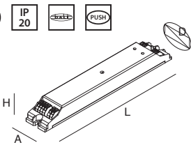
DALI REPEATER amplificatore per sistema DALI DALI REPEATER amplifier for DALI system
