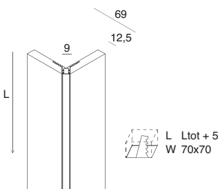
L-09 CORNER profilo lineare per spigolo esterno non installabile direttamente su muratura
