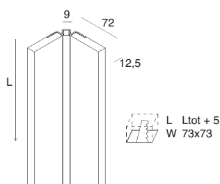
L-09 EDGE profilo lineare per spigolo interno
