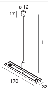
CAVO DI SOSPENSIONE (1 pz)
