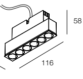
MODULO LED MICRO OTTICHE 200mA. Provisto di connettore rapido.
