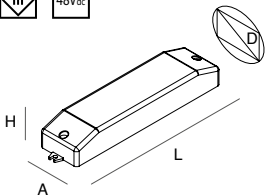
RIPETITORE PER OPTOISOLARE IL BUS DALI IN INGRESSO Dispositivo obbligatorio nel caso di utilizzo di CENTRALINA DALI, interfaccia pulsante 105926.99 o DALI repeater 18906.99. Vedi sezione Gestione Luce.
