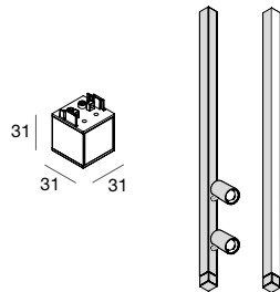
TESTATA DI SUPPORTO PER INSTALLAZIONE VERTICALE A PARETE Da prevedere obbligatoriamente nella parte inferiore del profilo se installato verticalmente a parete. SUPPORT END CAP FOR VERTICAL WALL MOUNTING To be provided compulsorily on the lower side of the profile, if mounted vertically on the wall.
