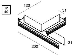
GIUNTO a T kit di giunzione incluso. Profili di chiusura da ordinare a parte. T JUNCTION junction kit included. Cover profiles to be ordered separately.
