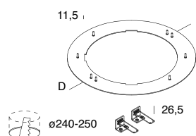
ADATTATORE PER NIK 32W per installazione in foro da incasso 240-250 mm, con molle.
