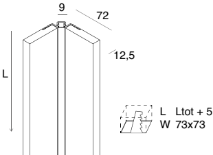
L-09 EDGE profilo lineare per spigolo interno
