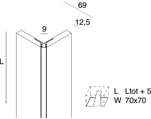
L-09 CORNER profilo lineare per spigolo esterno non installabile direttamente su muratura
