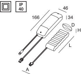
KIT DI ALIMENTAZIONE IN EMERGENZA Completo di connettori polarizzati per il collegamento dell'alimentatore. KIT FOR EMERGENCY Polarized connectors included.
